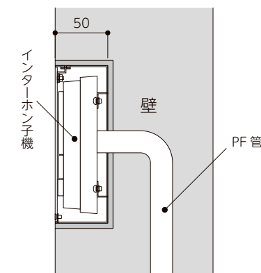
【MDP-3 参考施工図】
