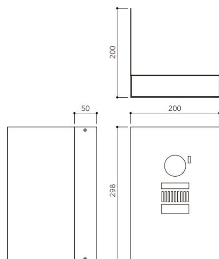
【MDP-4 参考施工図】
