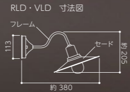
LED電球 7.9W防雨型付属 (一般電球 60W相当)
