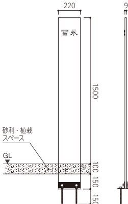
切文字 5mm 厚 ステンレスパーマライン
