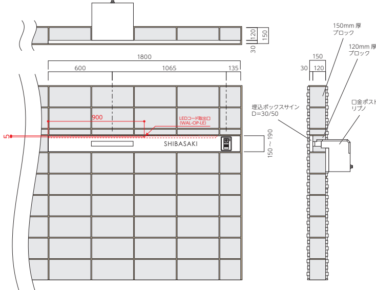
【参考施工図】 サイズ・文字位置・口金ポスト位置などはご注文内容によって異なります。
