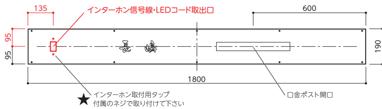
WAL-50 LED 付き サイズ・文字位置・口金ポスト位置などはご注文内容によって異なります。
