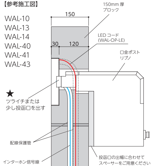
【参考施工図】
