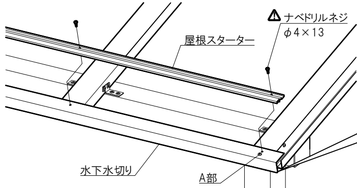
納まり詳細図
