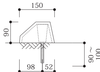
側面図
