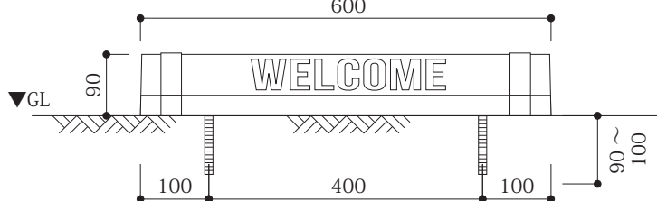
正面図
